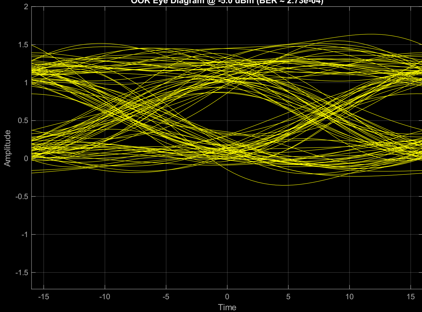
OOK Eye Diagram @ -5.0 dBm (BER \approx 2.73\text{e-}04 )
